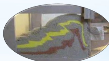
Modelos analógicos de deformación
